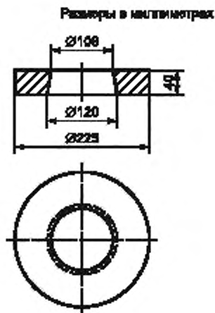
Рисунок 2 — Стальной раструб для обеспечения пригруза
